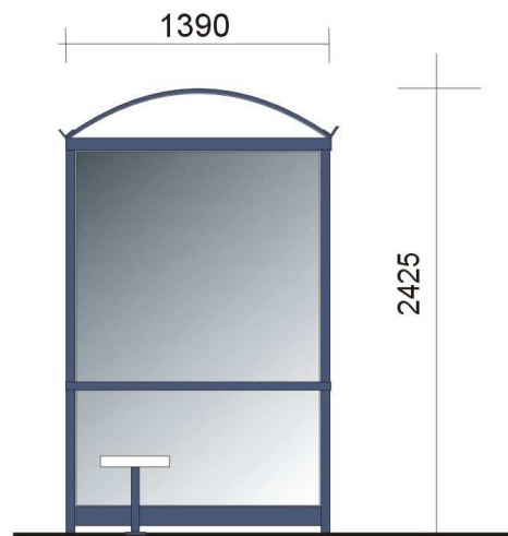
elewacja boczna pełne oszklenie
