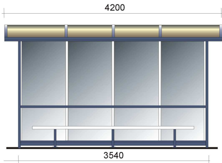
elewacja frontowa
