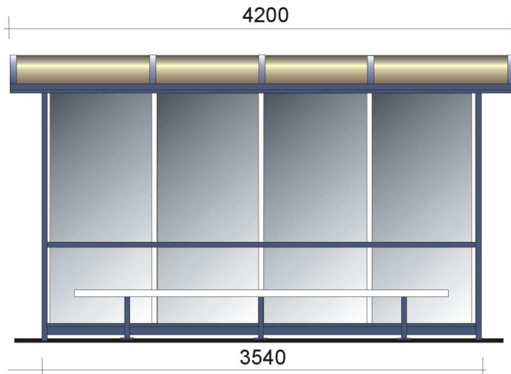
elewacja frontowa
